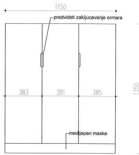
IZGLED O1 i O3 - ZATVOREN ORMAR
