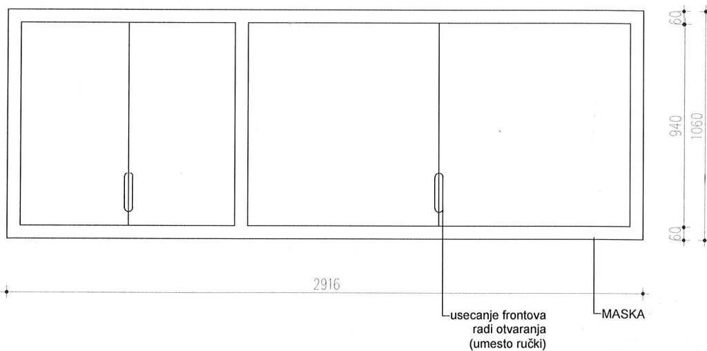
FRONT - ZATVOREN ORMAR
