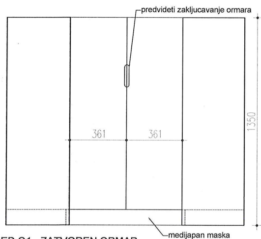
IZGLED O1 - ZATVOREN ORMAR
