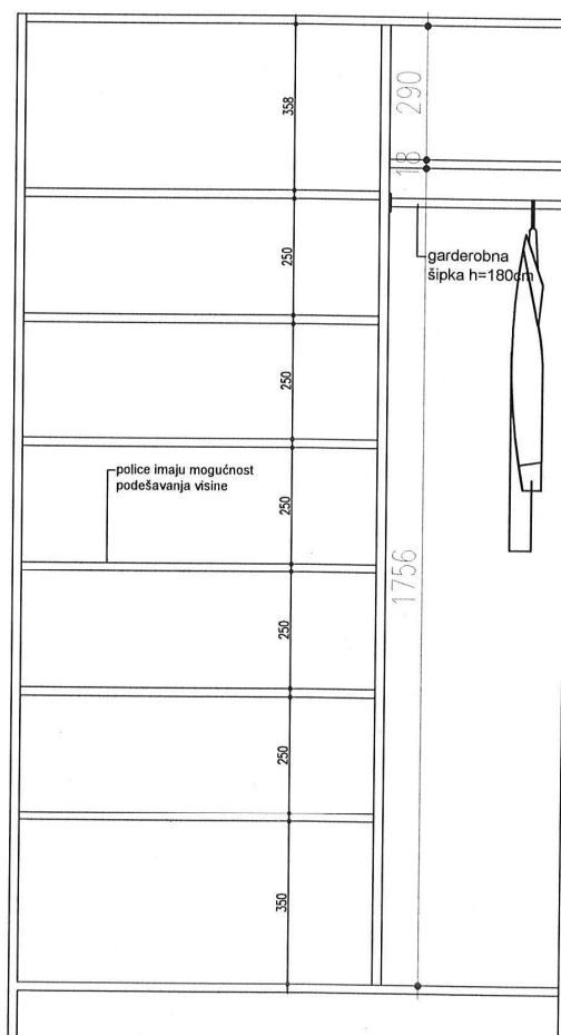
FRONT - OTVOREN ORMAR
