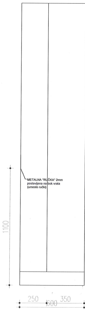
FRONT - ZATVOREN ORMAR
