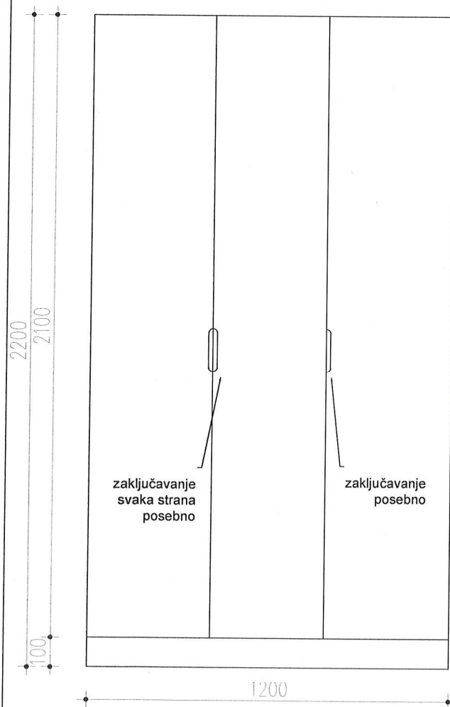
FRONT - ZATVOREN ORMAR
