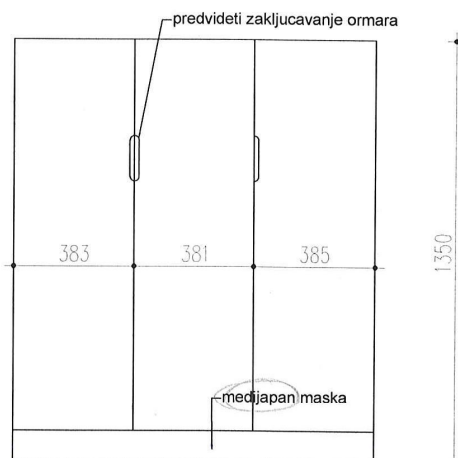
IZGLED O1 i O3 - ZATVOREN ORMAR
