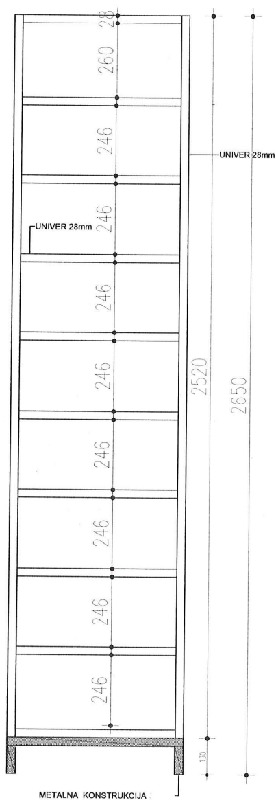
FRONT - OTVOREN ORMAR
